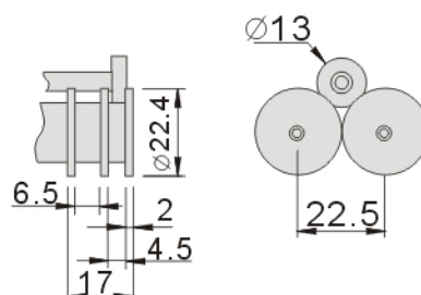
Détails galets deux gorges
