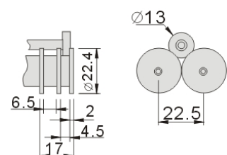
Détails galets deux gorges
