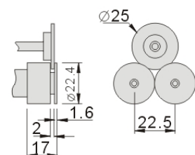
Détails galets une gorge
